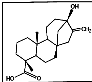
Figura 1. Esteviol.
