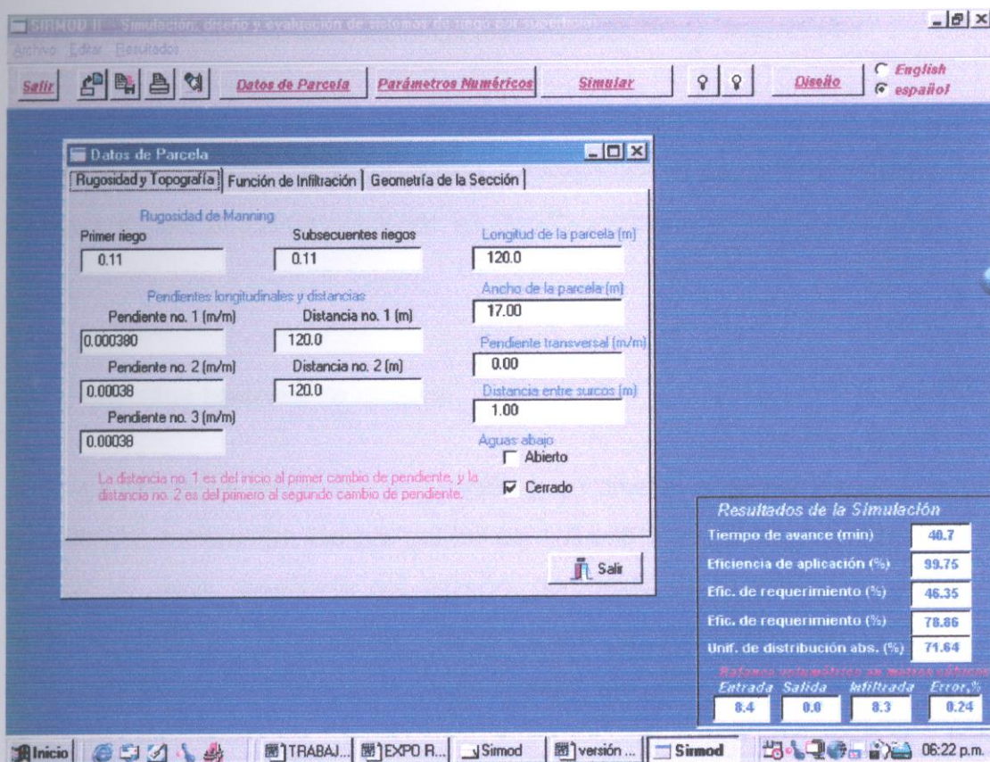
Figura 5.1. Pantalla de ajuste y diseño de SIRMOD que indica el ancho de melga, gasto unitario y pendiente.
