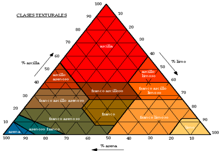
Figura 1. Clases Texturales
