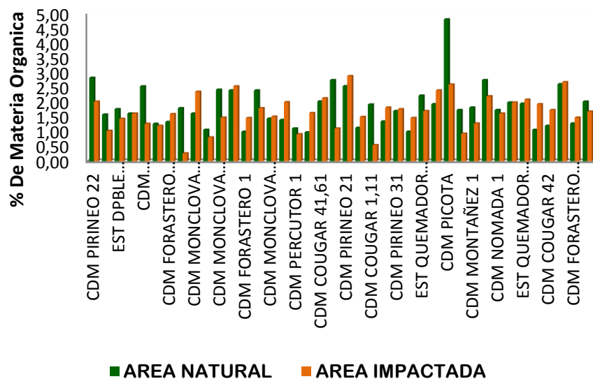
Figura 7. Porcentaje de M.O en cuadros de maniobras
