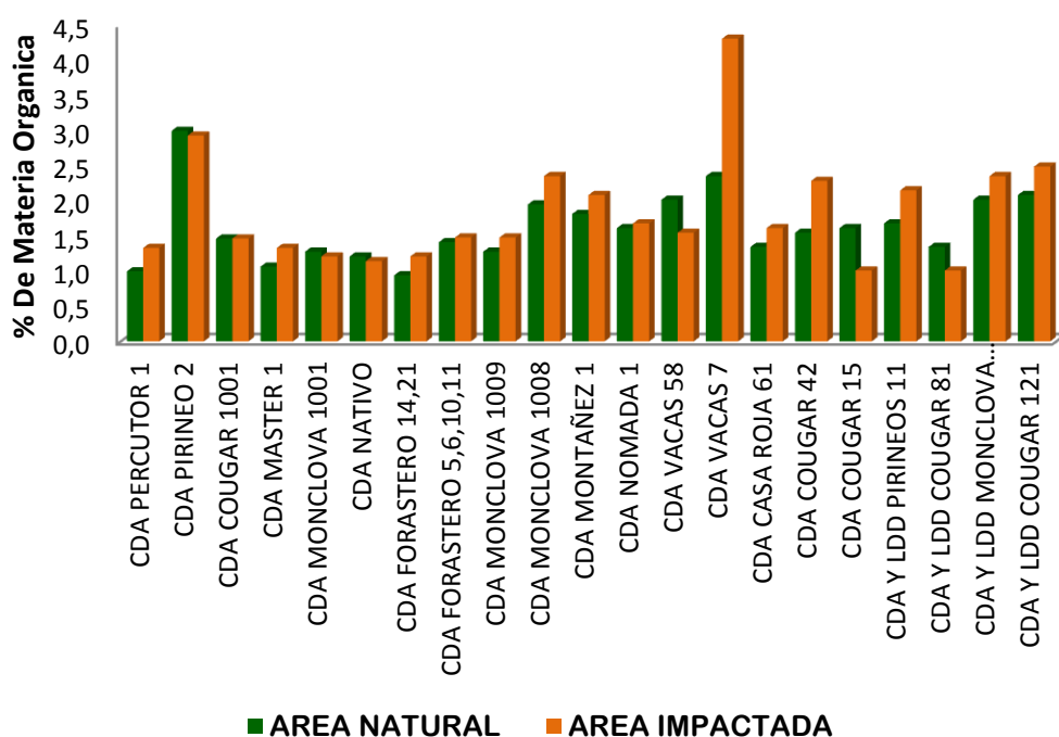
Figura 8. Porcentaje de M.O en caminos de acceso
