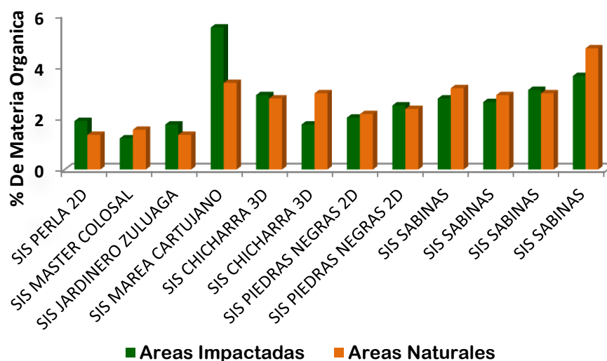
Figura 11. Porcentaje de M.O en áreas sísmicas
