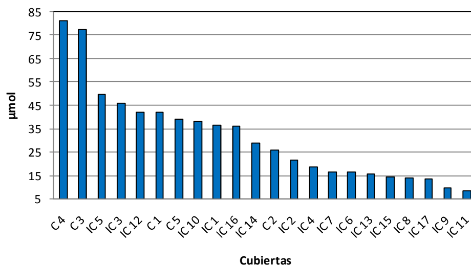
Fig. 4.3. Paso de la radiación UV para las 22 cubiertas.
