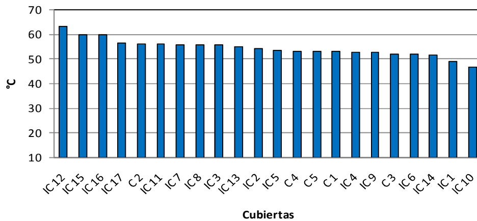
Fig.4.5. Temperatura dentro del microtúnel para las 22 cubiertas.
