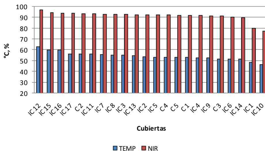
Fig.4.7. Comparación entre Temperatura (°C) y NIR ( %)
