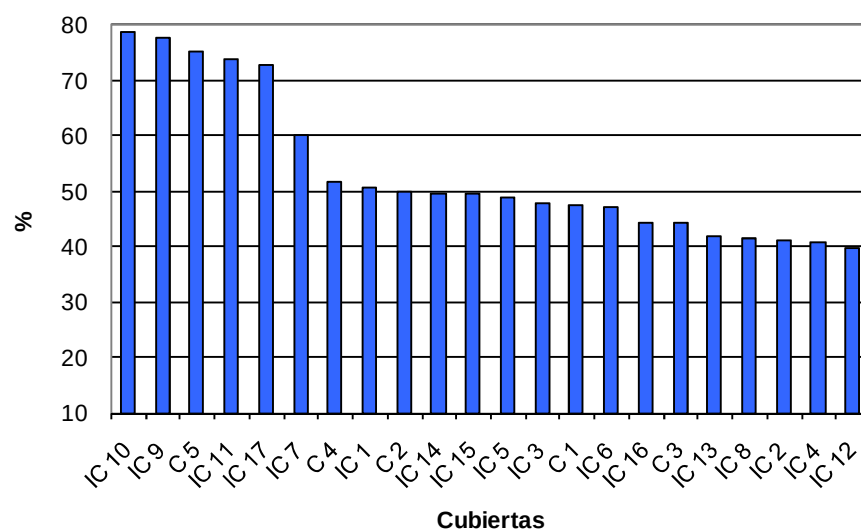
Fig.4.2. Porcentajes de la radiación difusa que dejan pasar las 22 cubiertas.
