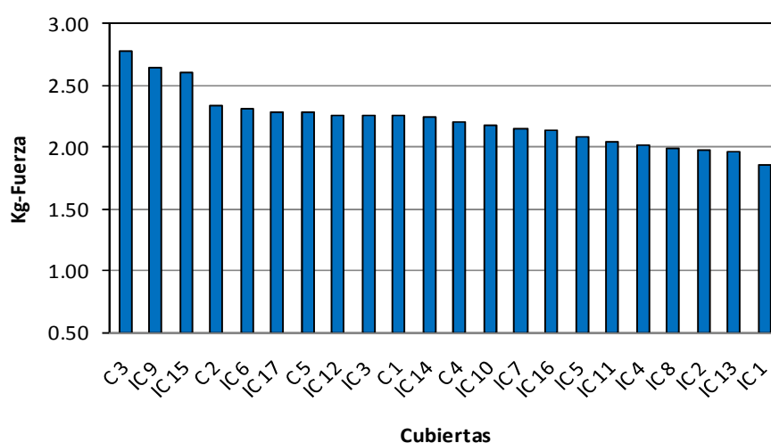
Fig. 4.1 Resistencia a punción de las diferentes cubiertas plásticas.
