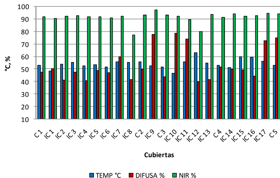
Fig. 4.6. Comparación de Temperatura,Difusa y NIR
