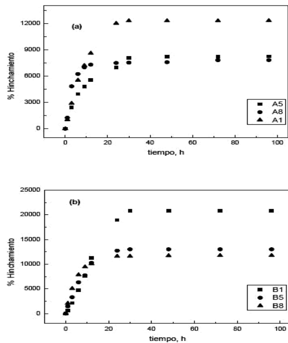
Figura 4. Hinchamiento de distintos hidrogeles en agua como función del tiempo y la cantidad de agentes entrecruzante: a) grupo A y b) grupo B (Katime et al. , 2004).
