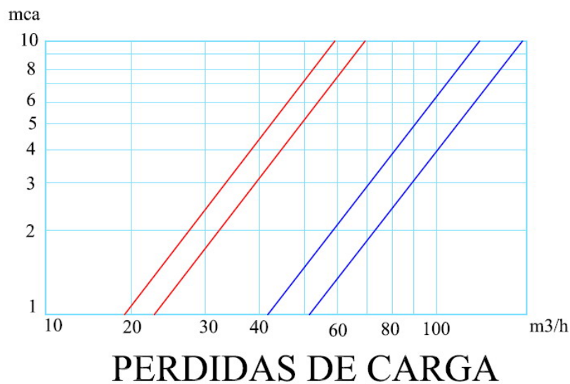
Figura 8. Grafica de Pérdidas de Carga.
