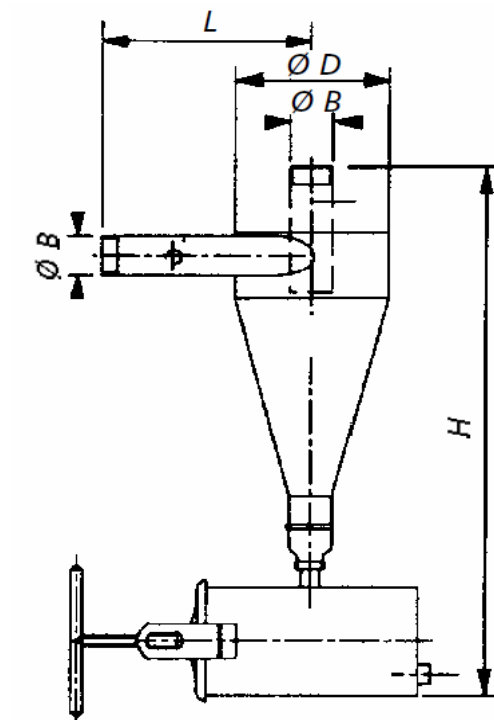
Figura 24. Principales dimensiones de los Hidrociclones.
